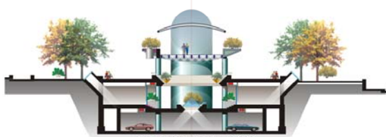
ԿՏՐՎԱԾՔ "7-7" Մ 1:400
