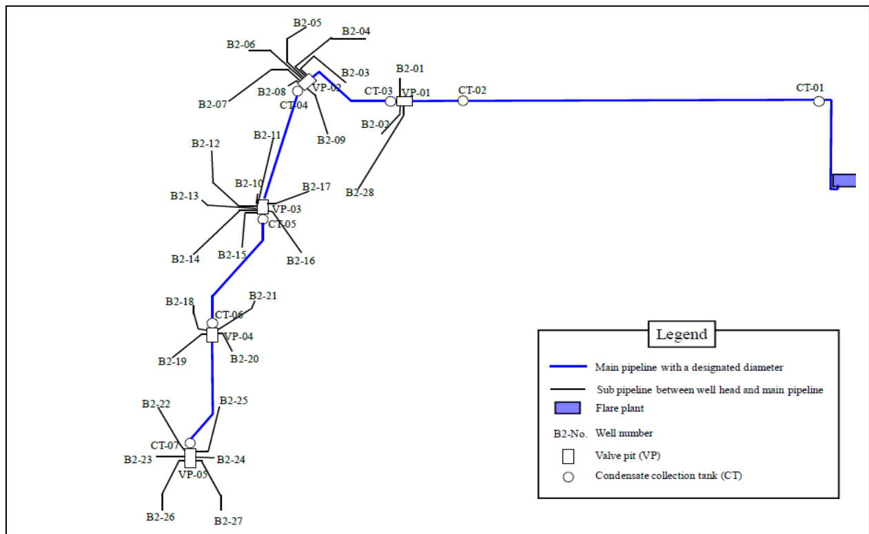
Նկար 5.2. Մեթանի կորզման 27 ուղղահայաց հորերի տեղաբաշխման սխեման Նուբարաշենի ԿԿԹ աղբույսի «Բոկ Բ-արևմտյան» հարթակում:
