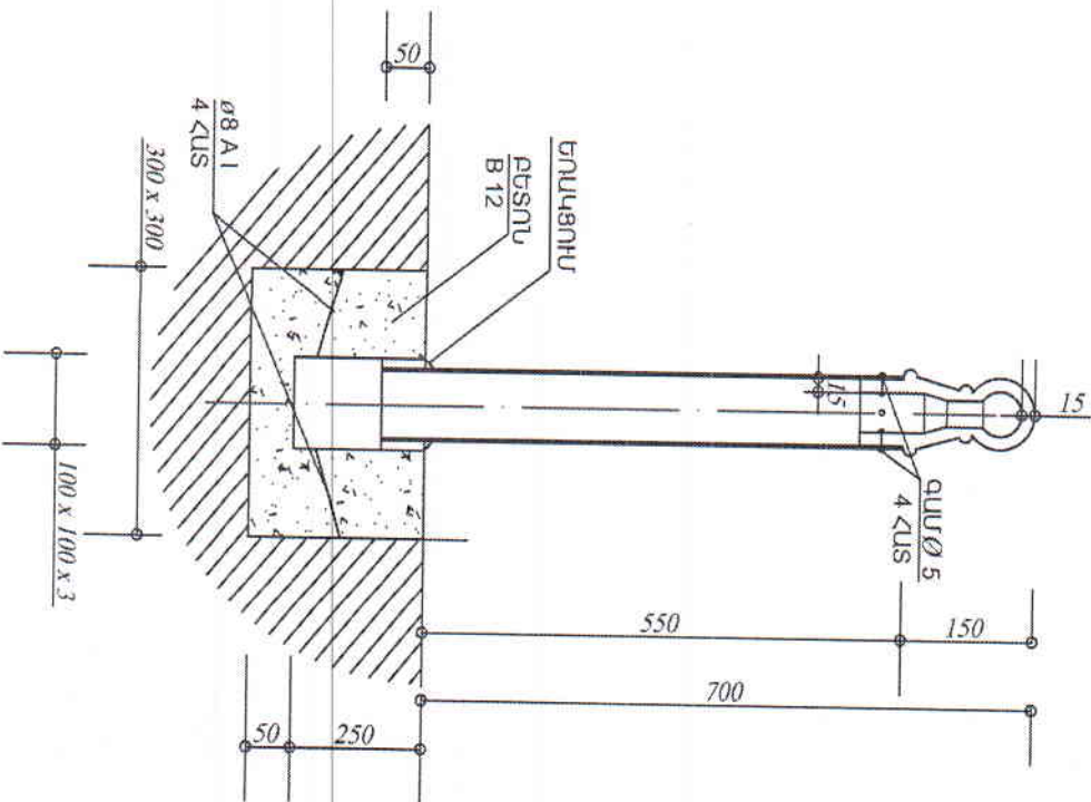
ԿՏՐԿԱԾՔ Մ 1:10
