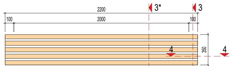
Նստարանի հատակագիծ U = 1:25
