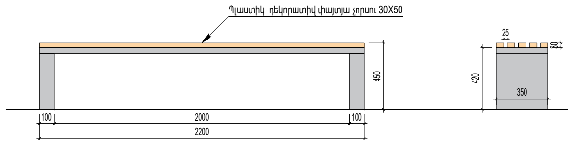
Նստարանի ձակատ ըստ Ա և Գ տեսքի U = 1:25
