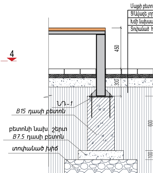
Կտրվածք 4.4 U = 1:25
