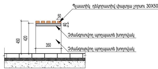
Նստարանի կտրվածք 3*-3* U = 1:25
