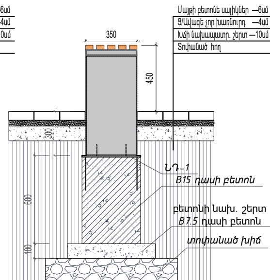
Կտրվածք 3-3 U = 1:25
