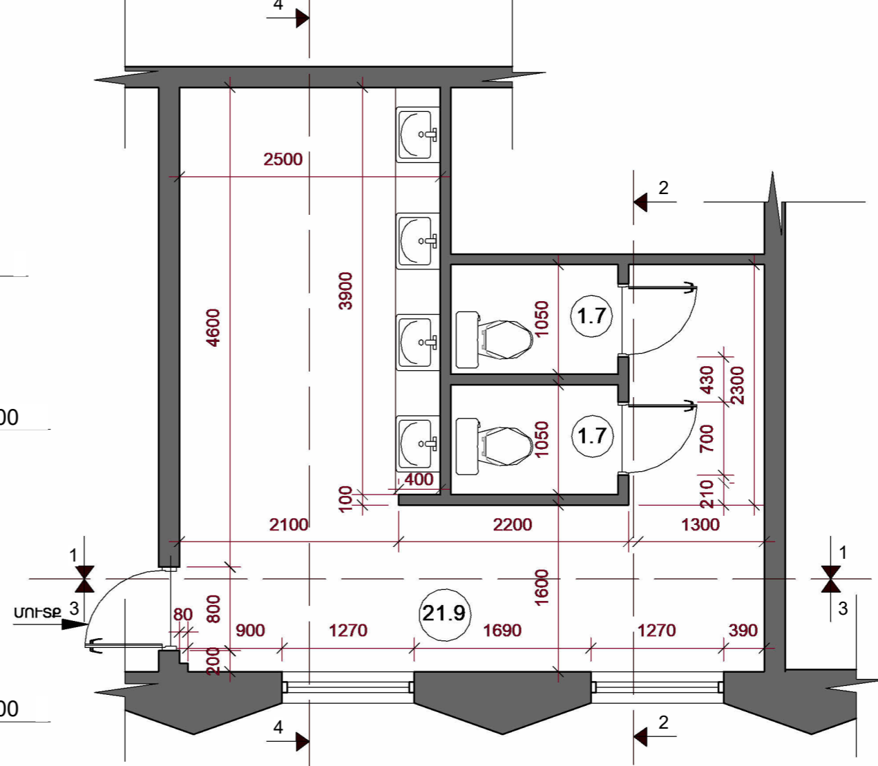
ՍԱՆՋԱՆԳՈՒՅՑԻ ԶԱՏԱԿԱԳԻԾ
