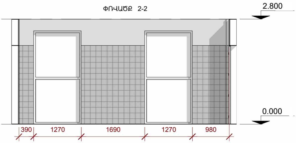
ՍԱՆՋԱՆԳՈՒՅՑԻ ԶԱՏԱԿԱԳԻԾ
