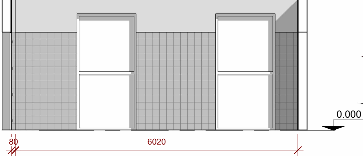
ՓՈՎԱԾԸ 4-4
