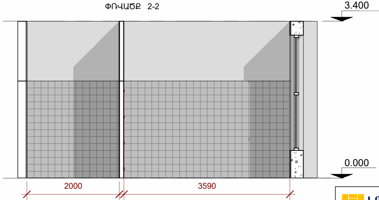
ՍԱՆՅԱՆԳՈՒՅՑԻ ԶԱՏԱԿԱԳԻԾ
