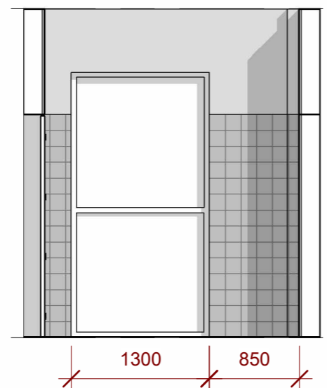
ՓՈՎԱԾԸ 6-6
