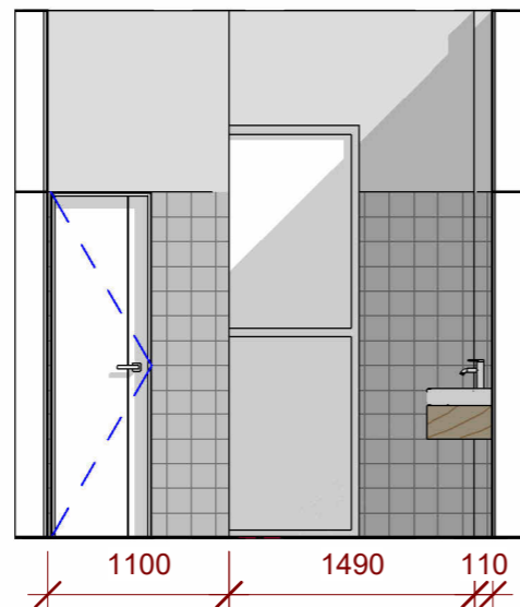
ՓՈՎԱԾԸ 4-4
