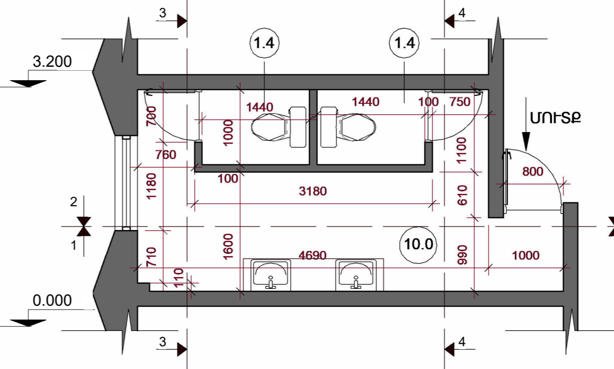
ՍԱՆՋԱՆԳՈՒՅՑԻ ԶԱՏԱԿԱԳԻԾ
