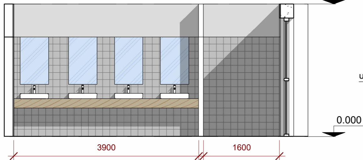
ՓՈՎԱԾԸ 4-4
