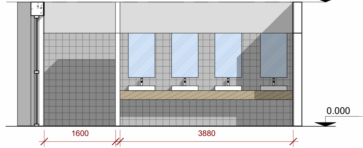
ՓՈՎԱԾԸ 2-2
