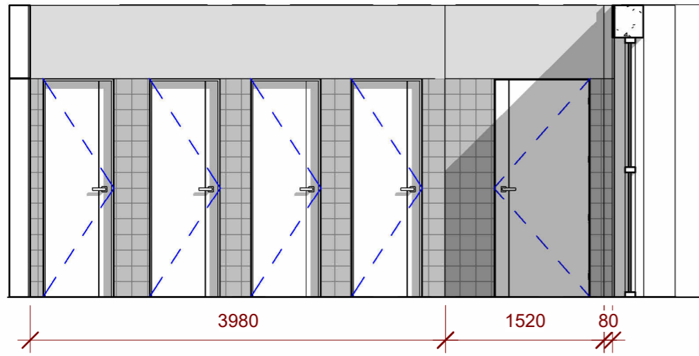
ՓՈՎԱԾԸ 1-1
