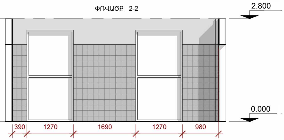
ՍԱՆՋԱՆԳՈՒՅՑԻ ԶԱՏԱԿԱԳԻԾ
