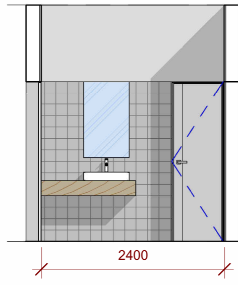
ՓՈՎԱԾԸ 6-6
