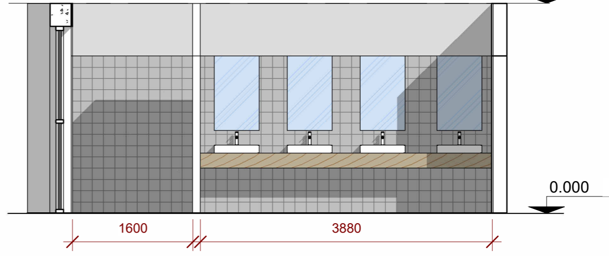
ՓՈՎԱԾԸ 2-2
