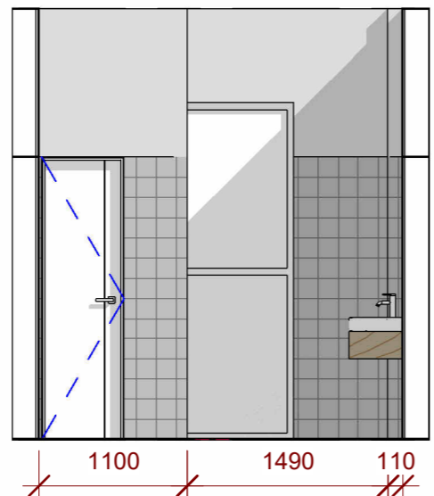
ՓՈՎԱԾԸ 4-4
