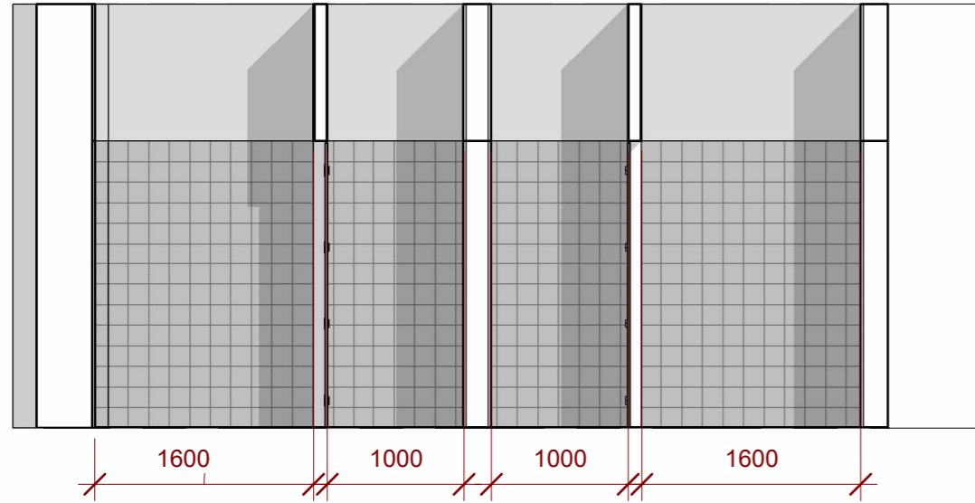
ՓՈՎԱԾԸ 1-1
