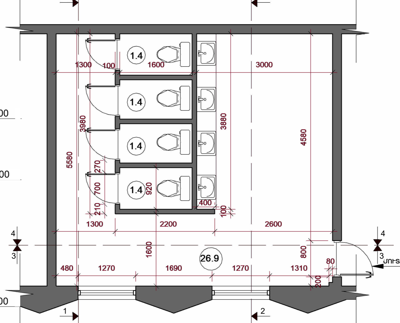
ՍԱՆՂԱՆԳՈՒՅՑԻ ԶԱՏԱԿԱԳԻԾ
