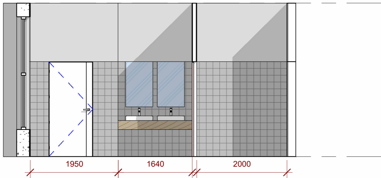
ՓՈՎԱԾԸ 1-1
